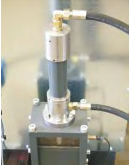
Endlagergedämpfter Füllzylinder und staubdichter Füllschacht Filling cylinder with damped end bearing and dust-tight filling shaft.
